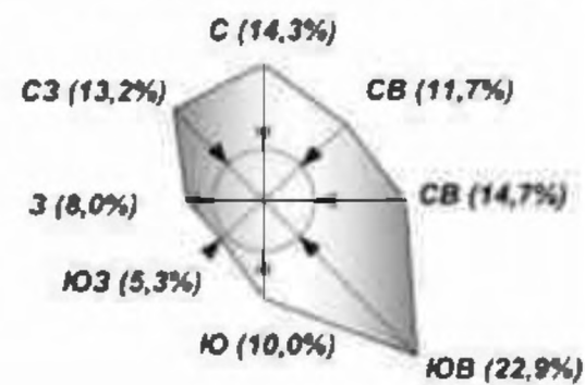
РОЗА ПОВТОРЯЕМОСТИ ВЕТРОВ
